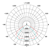
1390（隧道灯配光）
