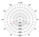
5390（90° 投射）
