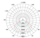
1390（隧道灯配光）
