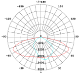
5340（40° 投射）
