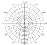
6001（60° 投射）
