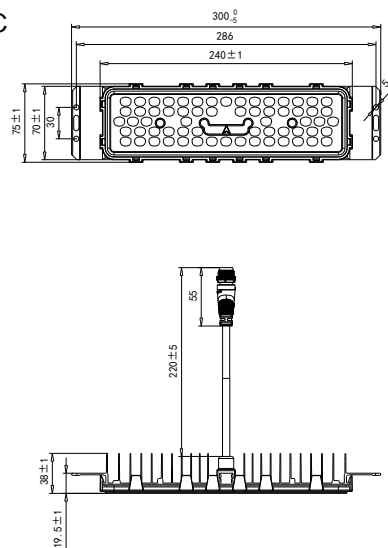
M16AS-CC
