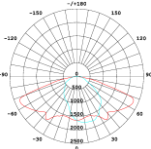
2360（60° 投射）
