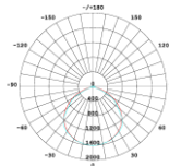
1310（朗伯型配光）
