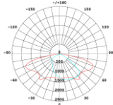
1325（25° 投射）
